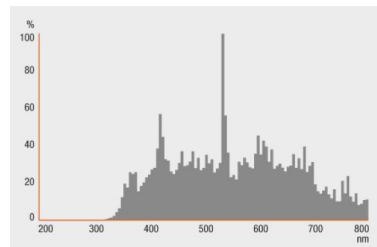
HAL PRO R50 30 W 230 V E14, HAL PRO R50 30 W 240 V E14
